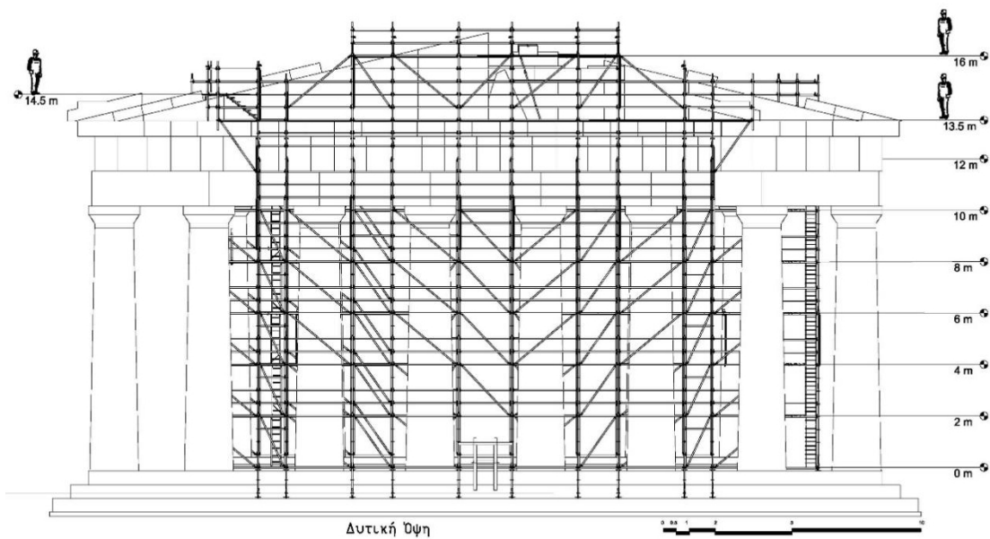
Εικ.4 Άποψη του ικρίωματος στην δυτική όψη του μνημείου.
