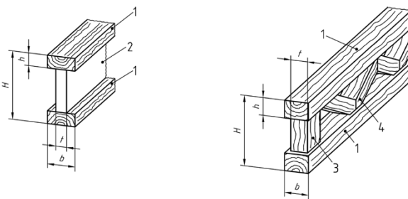
Εικ.6 Ξύλοδοκοί
