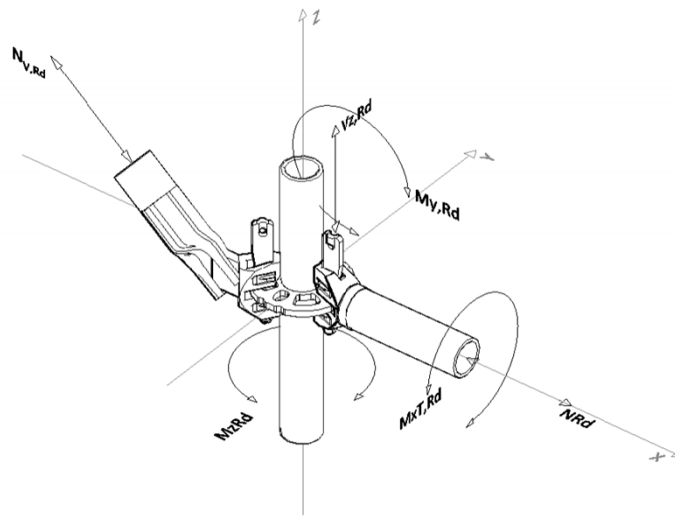
Εικ.7 Απεικόνιση των δυνάμεων – ροπών στον κόμβο του συστήματος τύπου ροζέτα (ring system ή ringlock)
