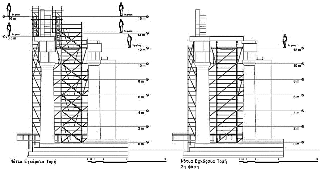
Εικ.3 Τομή στο νότιο πτερό με ορατή την νότια πλευρά του ικρίωματος (1 η και 2 η φάση εργασιών, με τις στάθμες των δαπέδων εργασίας)
