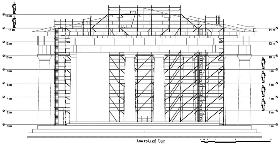
Εικ.5 Άποψη του ικρίωματος από την ανατολική πλευρά του Οπισθοναού.
