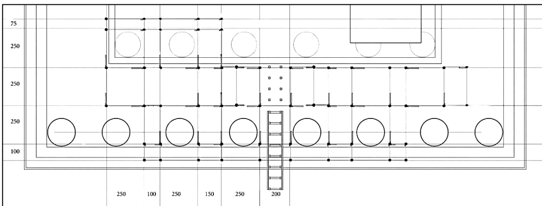
Εικ.2 Ενδεικτικός κάνναβος θέσης ορθοστατών
